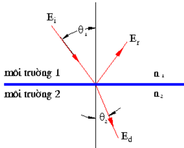
Hình 2.10. Quá trình truyền của tia bức xạ.
