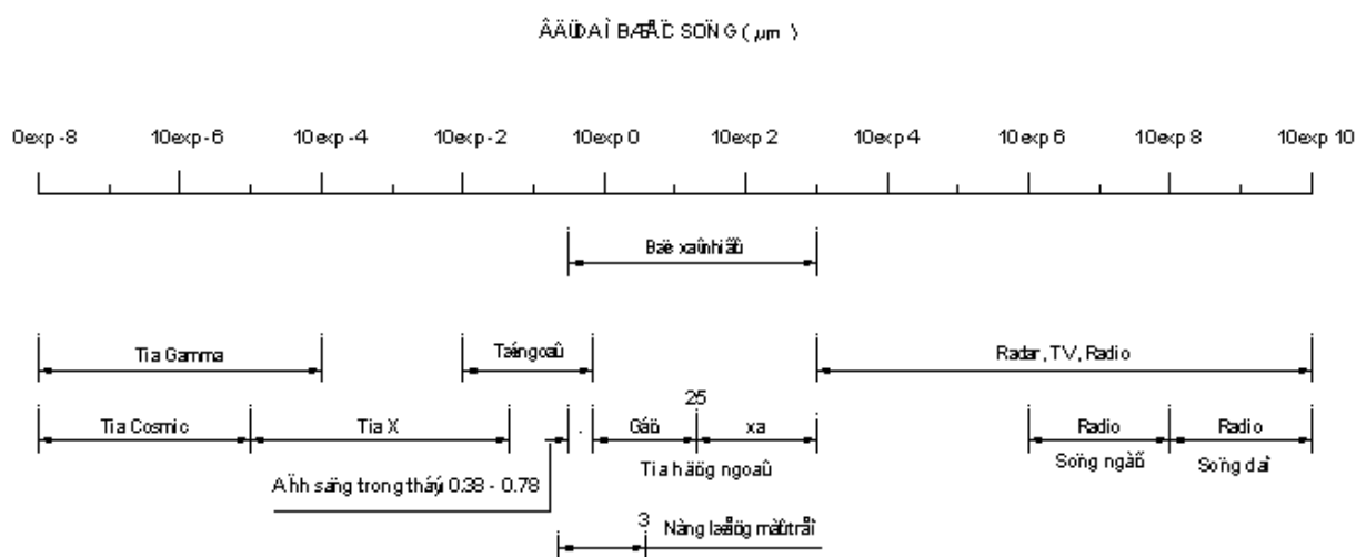
Hình 2.1 Dải bức xạ điện từ
