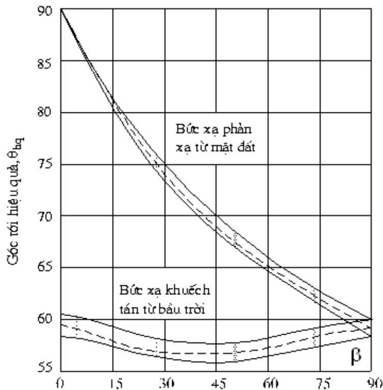
Hình 2.12. Góc tới hiệu quả của tán xạ đẳng hướng và bức xạ phản xạ từ mặt đất trên mặt phẳng nghiêng.
