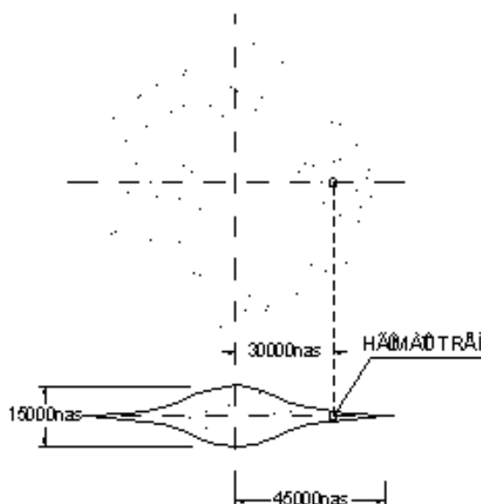
Hình 1.1. Ngân hà và hệ mặt trời
